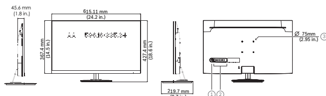
图片 1: 高性能LED监视器 (27英寸) 尺寸
