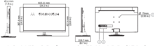
Şek. 1: Yüksek Performanslı LED Monitörün (27 inç) Boyutları
