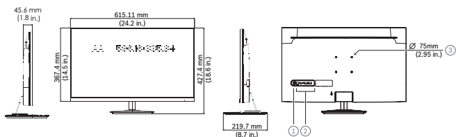
Fig. 1: Dimensões do monitor de LED de alto desempenho (27 pol.)
