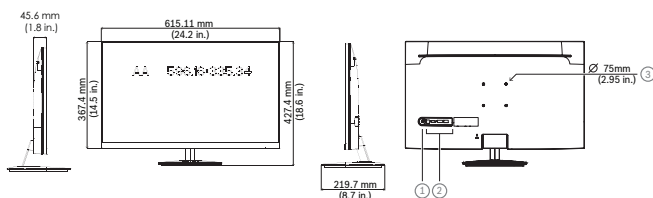
Fig. 1: Dimensioni monitor LED ad alte prestazioni (27 pollici)
