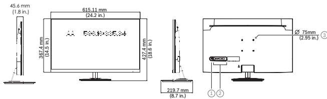
Fig. 1: Monitor LED de alto rendimiento de dimensiones (27 pulg.)
