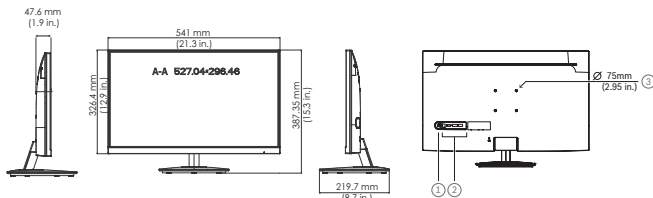
Fig. 1: Dimensioni monitor LED ad alte prestazioni (24 pollici)
