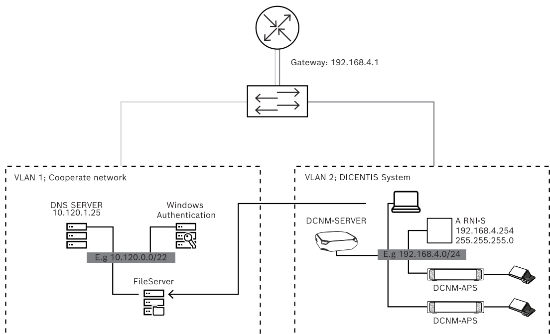
圖片 5.2: 系統圖
