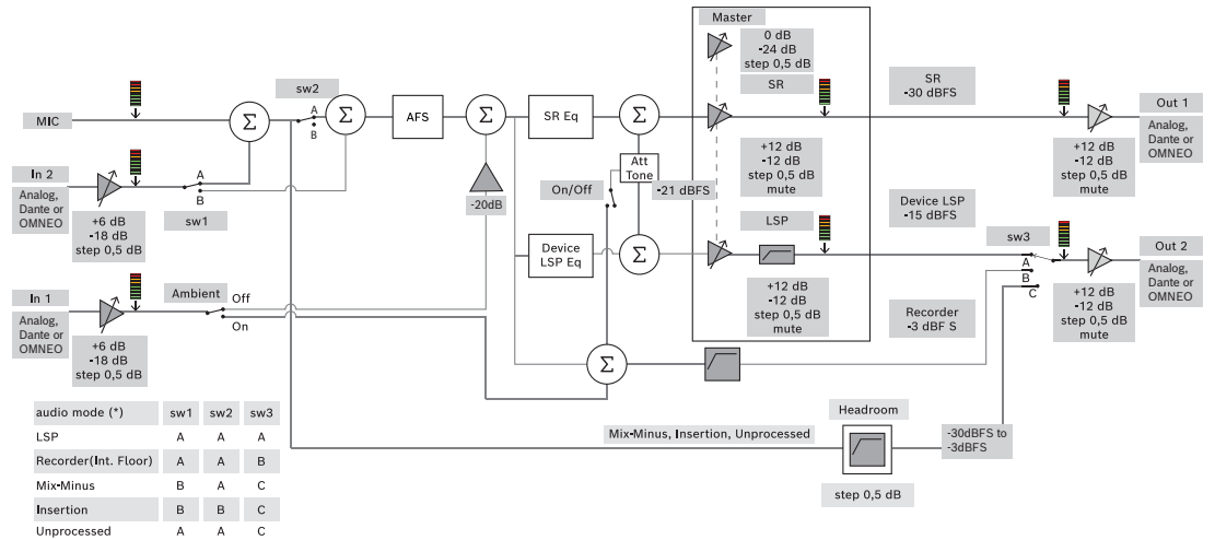
圖片 5.5: 音訊路由設定
