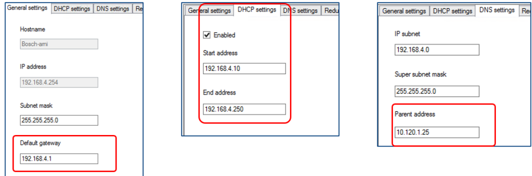
圖片 5.3: 具有 ARNI 的系統設置
