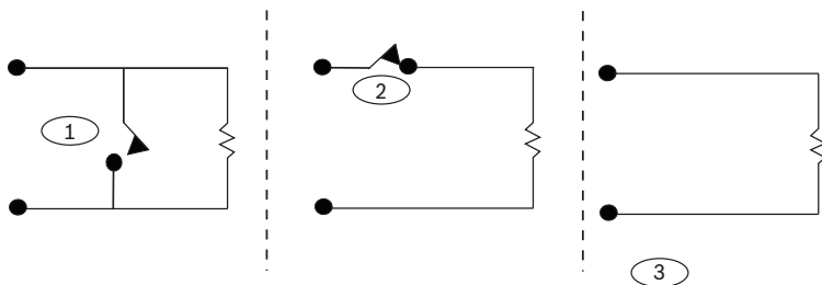
Figura 16.1: Opción de resistencia de RFL simple
