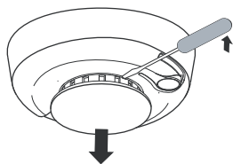
Figura 12.2: Extracción de la tapa del detector
