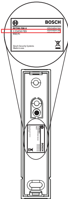
Figura 3.3: Ejemplo de adhesivo de ID de RF
