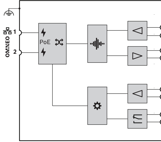
İşlev ve bağlantı şeması
