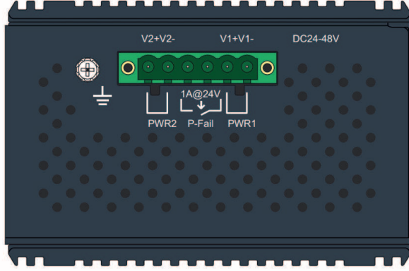
Üstteki panel bağlantıları
