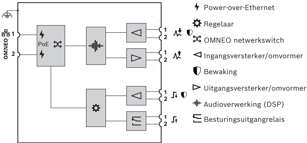
Functie- en aansluitingsdiagram
