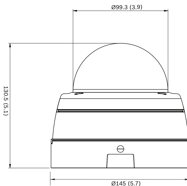
fig. 1: Dimensioner mm (inch)
