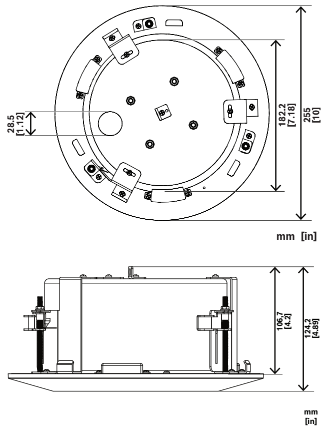
Fig. 1: NDA-8002-PLEN IR
