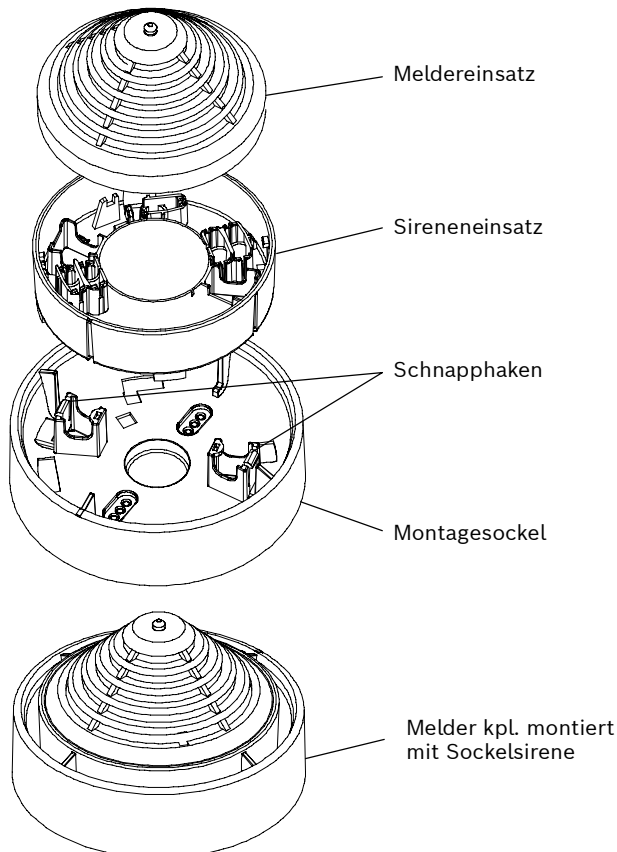
Bild 3: Montagereihenfolge
