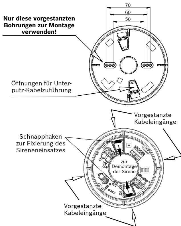
Bild 2: Installationsdetails
