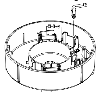
Bild 4: Melderverriegelung
