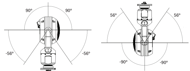
Afb. 1: Kantelbereik van MIC IP fusion 9000i-camera
