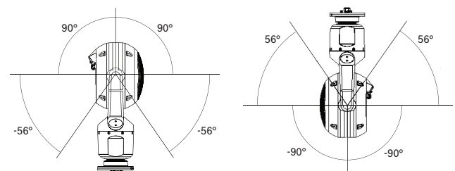
Abb. 1: Neigebereich der MIC IP fusion 9000i-Kamera
