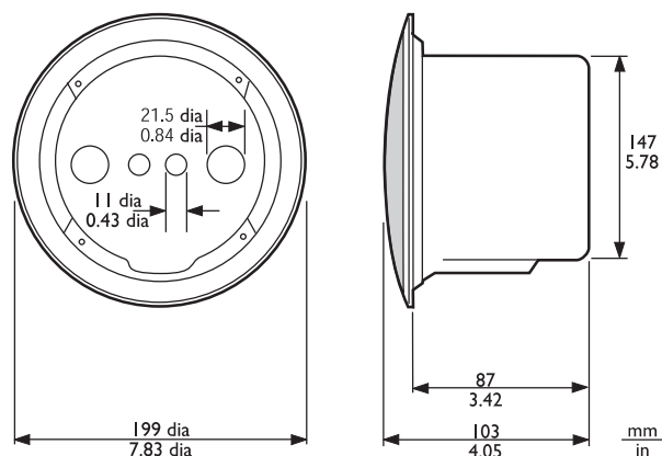
Hình 8: Kích thước của bộ vỏ nhôm chôn chấu LBC3090/01 + LBC3080/01 tính theo mm (in)
