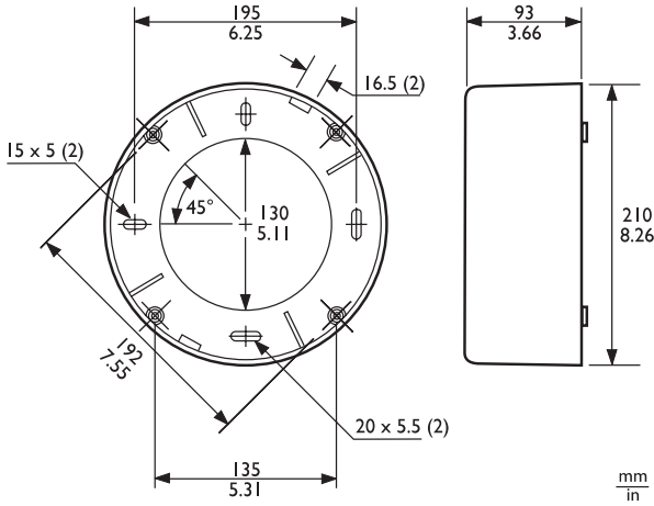
Şek. 7: mm (inç) cinsinden boyutlar
