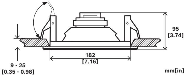
Şek. 2: mm (inç) cinsinden boyutlar
