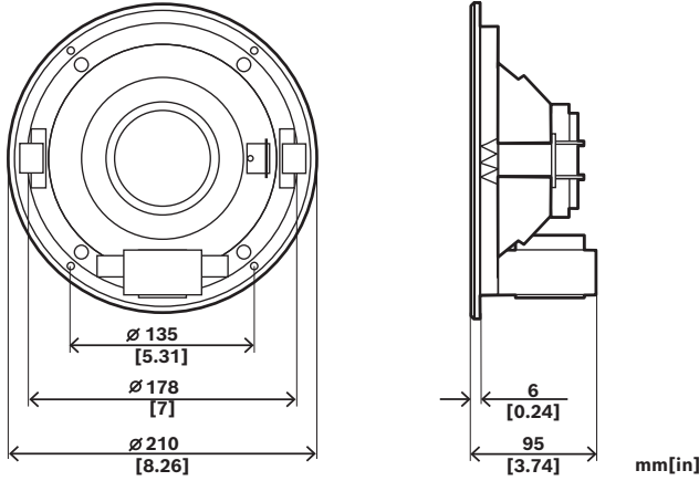
Şek. 1: mm (inç) cinsinden boyutlar
