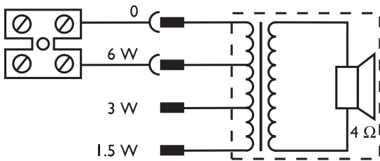
Şek. 3: Devre şeması
