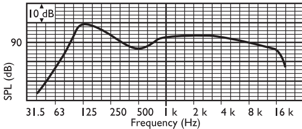
Şek. 4: Frekans tepkisi
