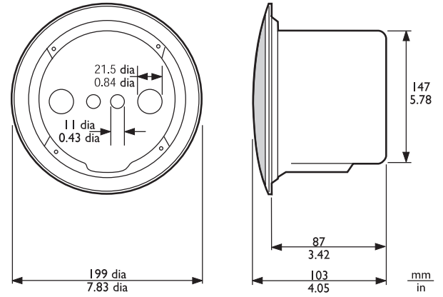
Şek. 8: LBC3090/01 + LBC3080/01 yangın koruma kapağı düzeneği mm (inç) cinsinden boyutlar
