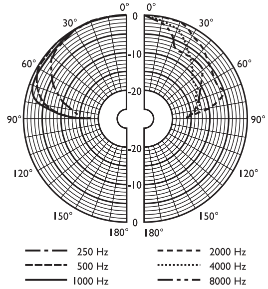
Şek. 5: Kutup şeması (pembe gürültüyle ölçülmüştür)
