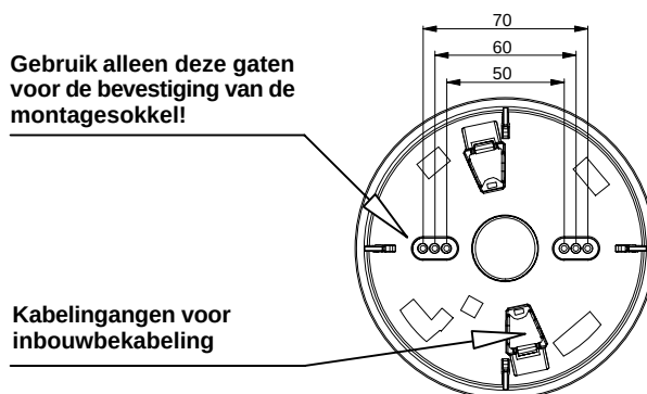
Afbeelding 2: montagedetails
