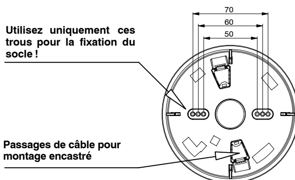
Figure 2 : détails d'installation
