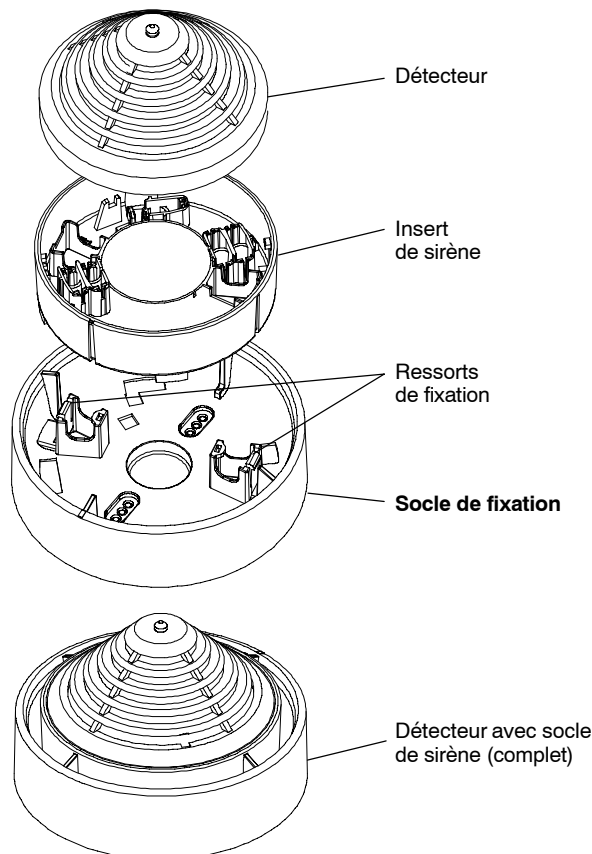
Figure 3 : ordre de montage
