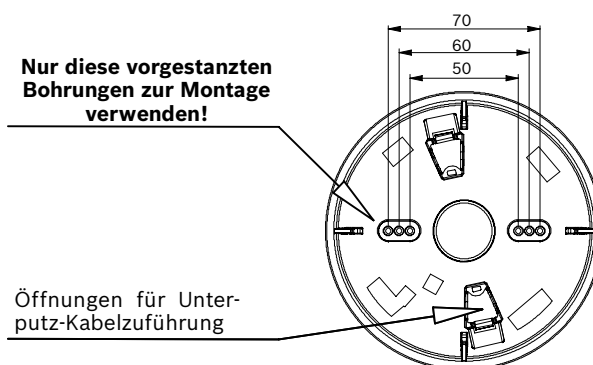
Bild 2: Installationsdetails
