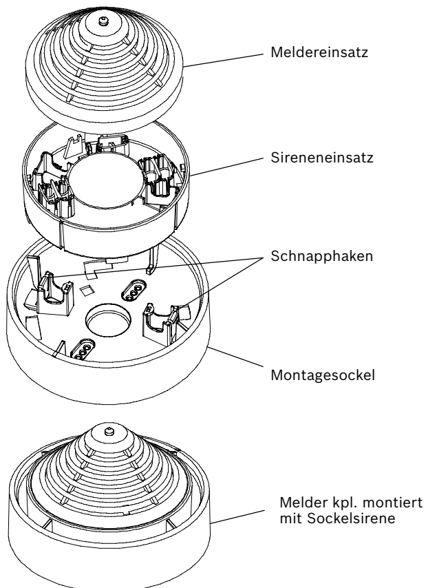
Bild 3: Montagereihenfolge
