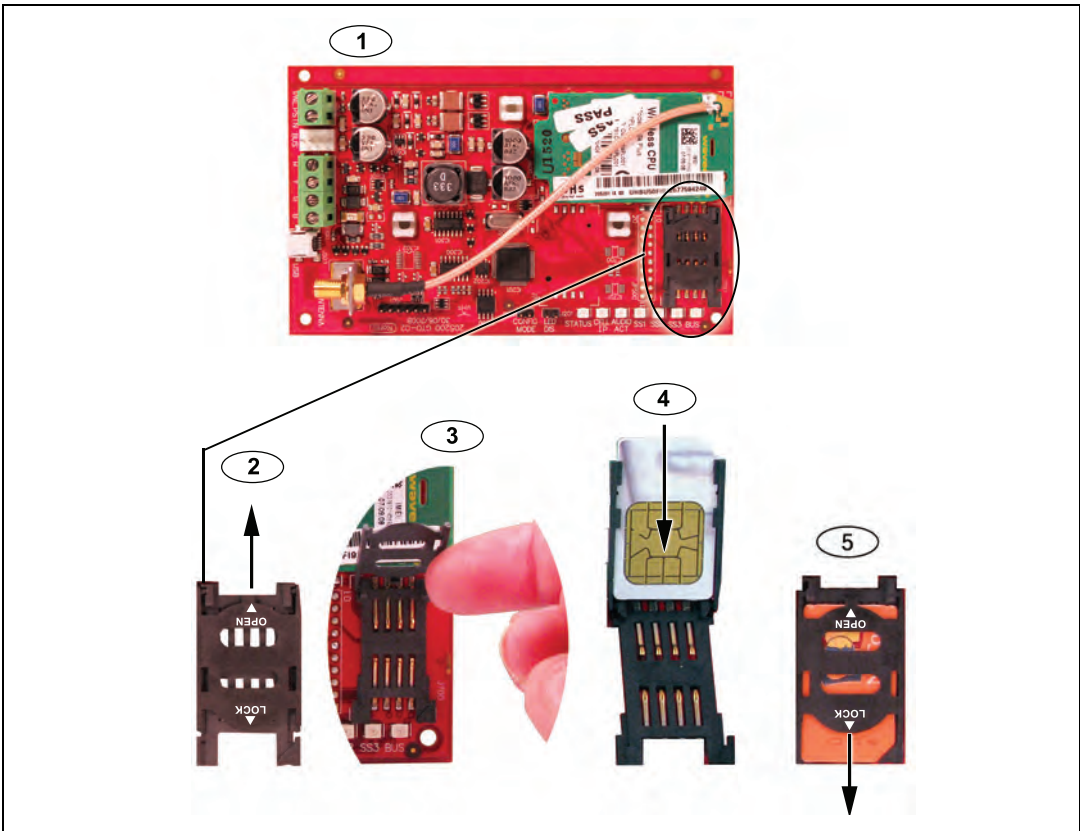
Afbeelding 3.1 Overzicht SIM-kaart en kaarthouder
