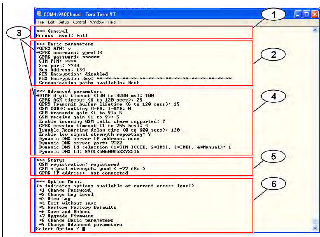
Afbeelding 4.3 USB-hoofdmenu
