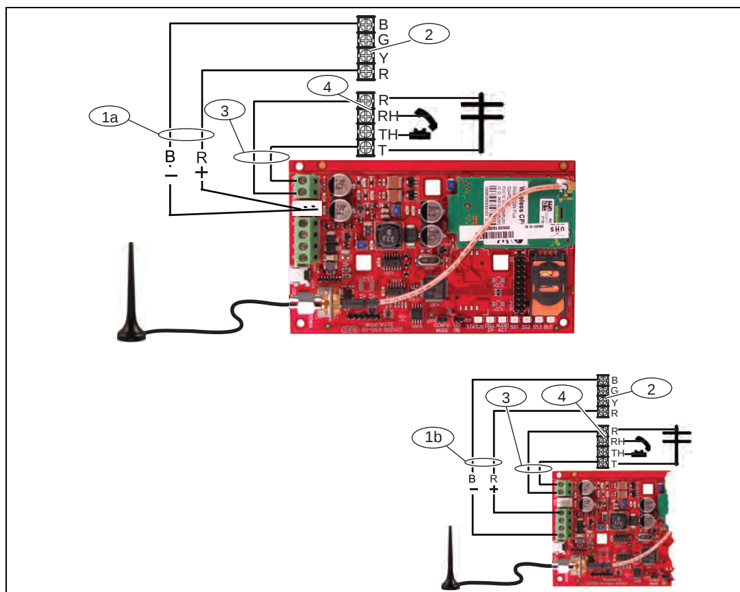
Afbeelding 3.4 Verbindingen voor de modus PSTN (contact-ID) via GSM
