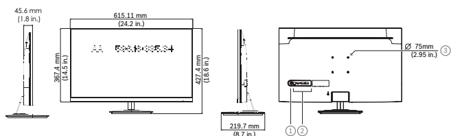
Afb. 2: Afmetingen hoogwaardige LED-monitor (27 inch)
