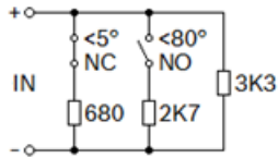
Fig. 4: Control de la posición de la compuerta de sobrepresión mediante resistencias triples
