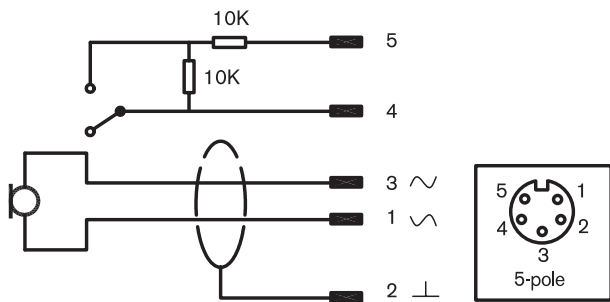
电路图
