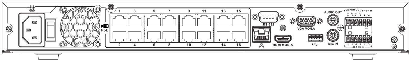
圖 2: DIVAR 3000 network 後方面板 (16 PoE)
