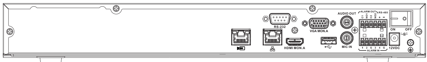
圖 1: DIVAR 3000 network 後方面板 (無 PoE)
