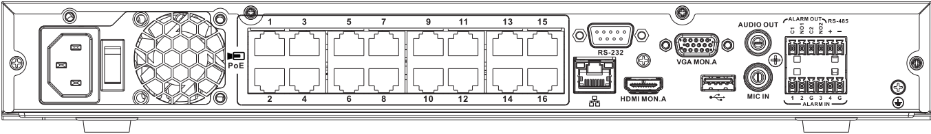
图片 2: DIVAR 3000网络后面板(16 PoE)
