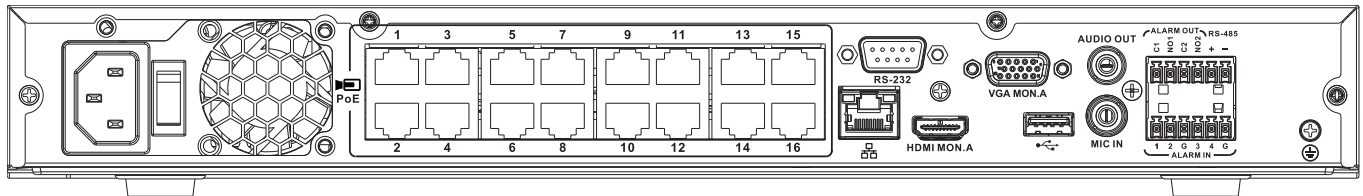
Şek. 2: DIVAR 3000 network arka panel (16 PoE)
