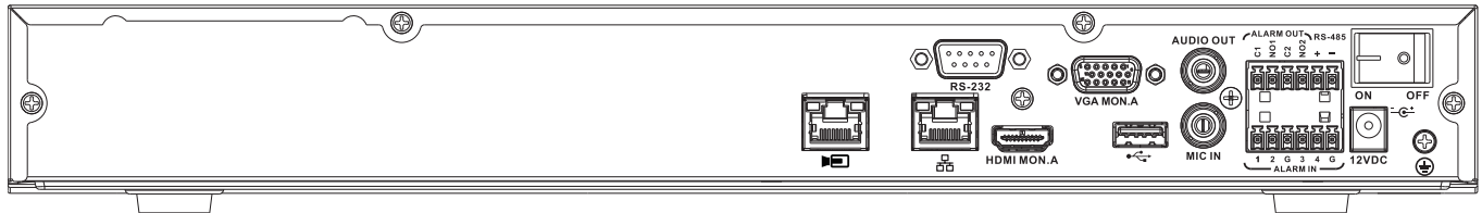
Şek. 1: DIVAR 3000 network arka panel (PoE yok)
