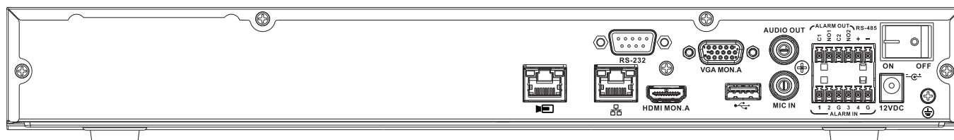
Рис. 1: Задняя панель DIVAR network 3000 (без PoE)
