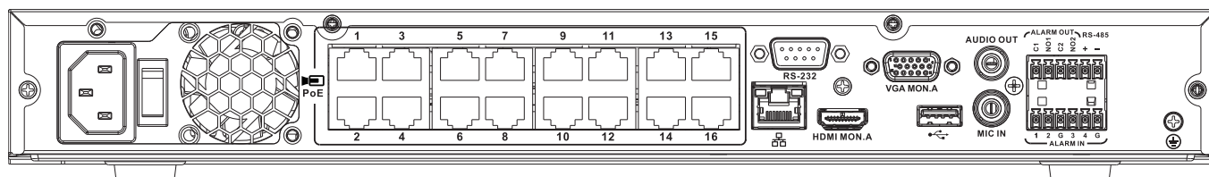
Rys. 2: Panel tylny rejestratora sieciowego DIVAR network 3000 (16 PoE)
