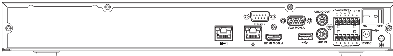
Rys. 1: Panel tylny rejestratora sieciowego DIVAR network 3000 (bez PoE)
