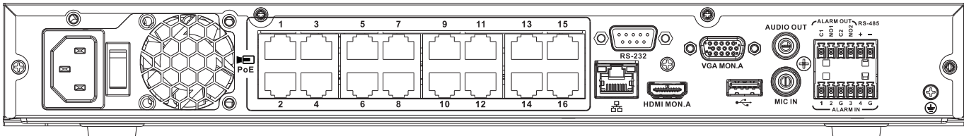
DIVAR 3000 网络后面板(16 PoE)
