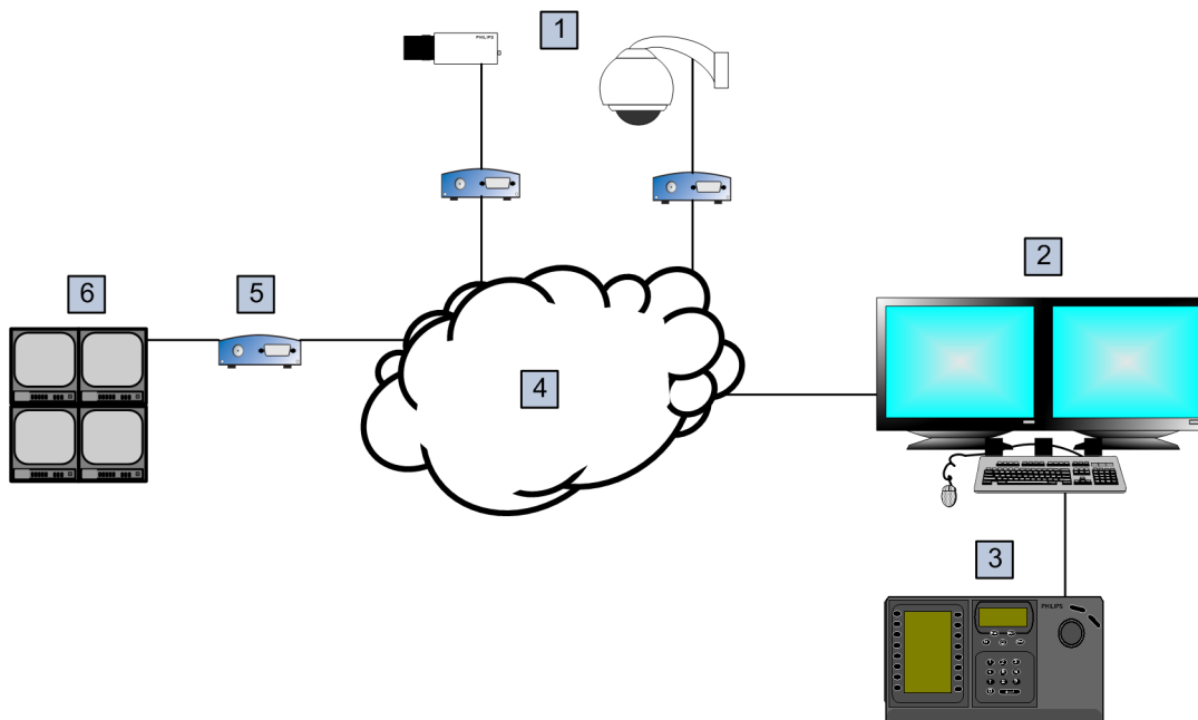
Σχήμα 5.1: Σενάριο 1: Πληκτρολόγιο IntuiKey της Bosch συνδεδεμένο με σταθμό εργασίας του Bosch Video Management System
