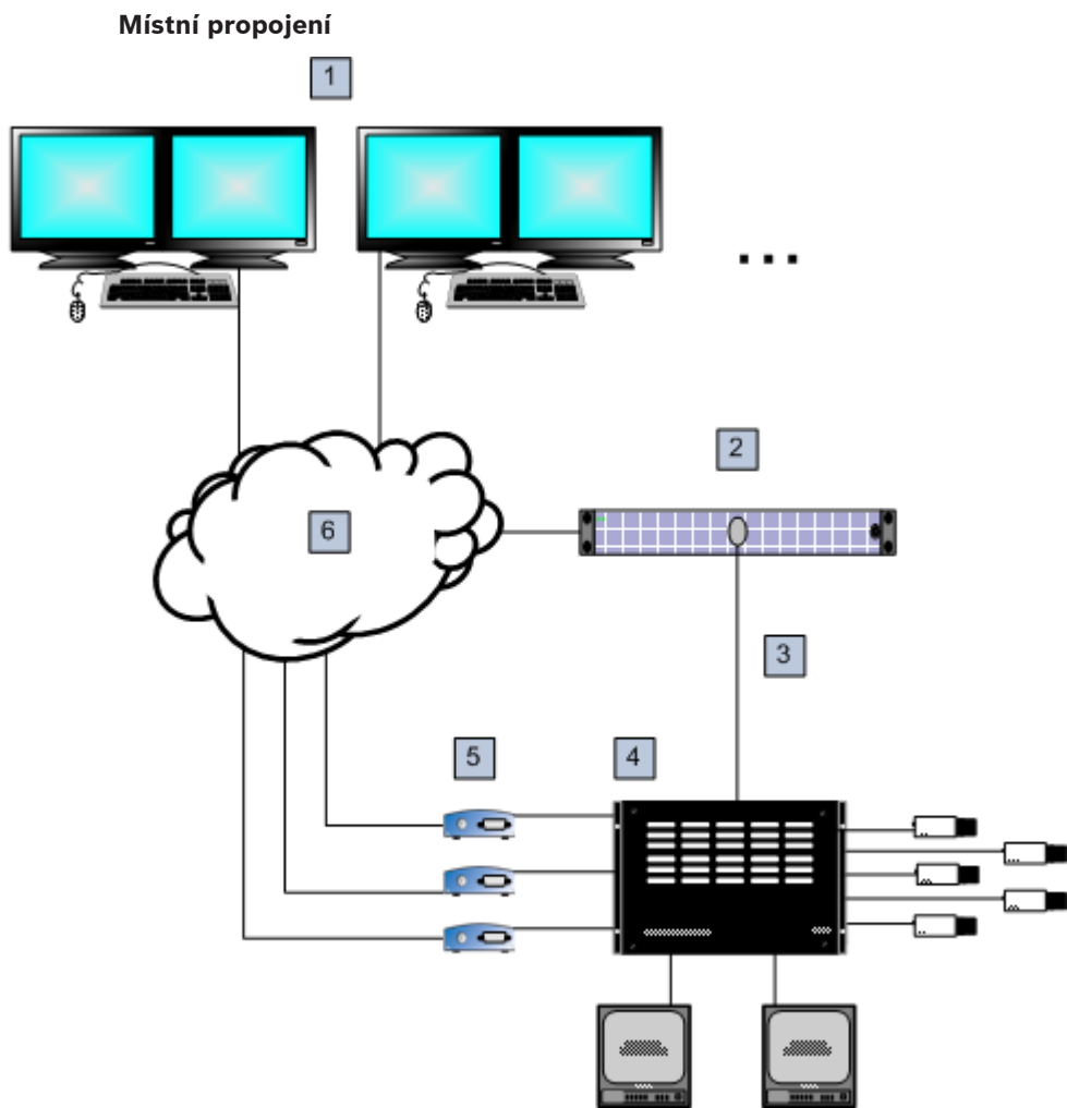
Obrázek 5.1: Místní propojení systému Bosch Video Management System s maticovým přepínačem Bosch Allegiant
