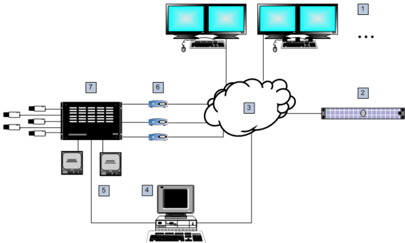
Obrázek 5.1: Vzdálené propojení systému Bosch Video Management System s maticovým přepínačem Bosch Allegiant
