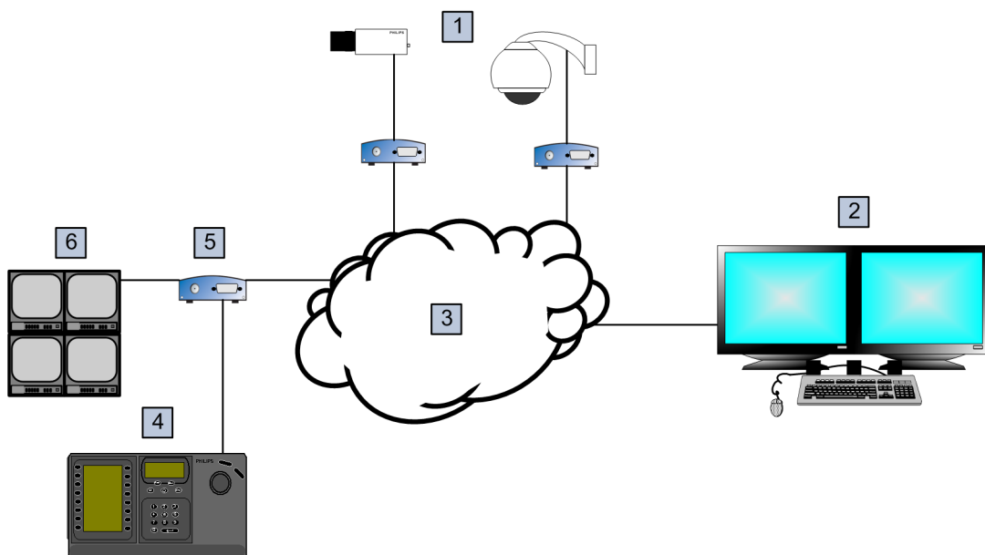
Obrázek 5.1: Scénář 2: Klávesnice Bosch IntuiKey připojená k dekodéru
