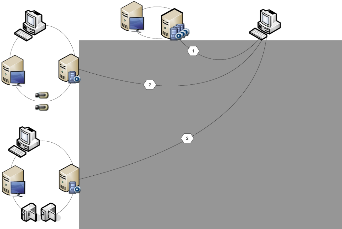
그림 4.1: 엔터프라이즈 시나리오 1
