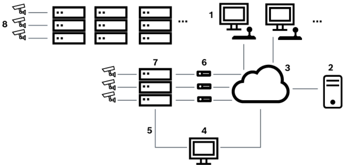
Рис. 6.5: Система Bosch Allegiant, расширенная за счет спутниковых коммутаторов
