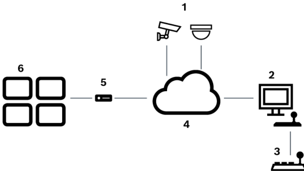
Figura 6.1: Cenário 1: Teclado IntuiKey da Bosch ligado a uma estação de trabalho Bosch Video Management System
