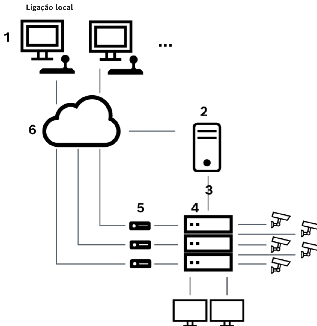
Figura 6.3: Ligação local do Bosch Video Management System a um computador matricial Allegiant Bosch
