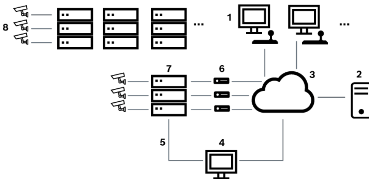
Figura 6.5: Sistema Allegiant Bosch ampliado com comutadores Satélite
