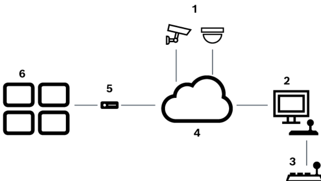
Attēls 6.1: 1. scenārijs: Bosch IntuiKey tastatūra, kas savienota ar Bosch Video Management System darbstaciju
