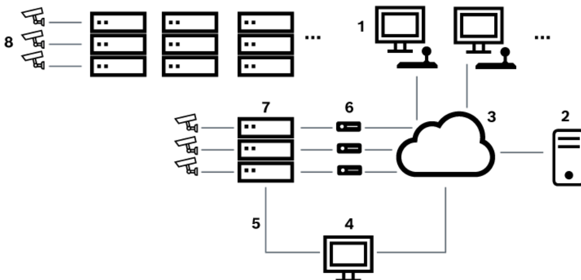
Attēls 5.5: Bosch Allegiant sistēma, kas paplašināta ar satelīta slēdžiem
