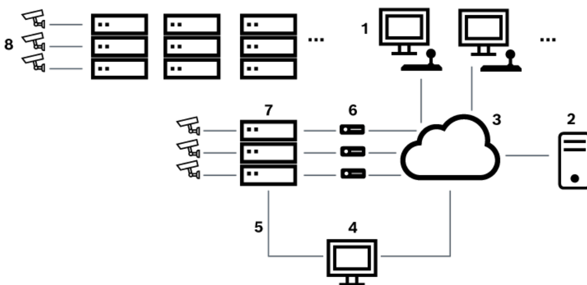
Rysunek 5.5: System Bosch Allegiant rozbudowany o przełączniki satelitarne
