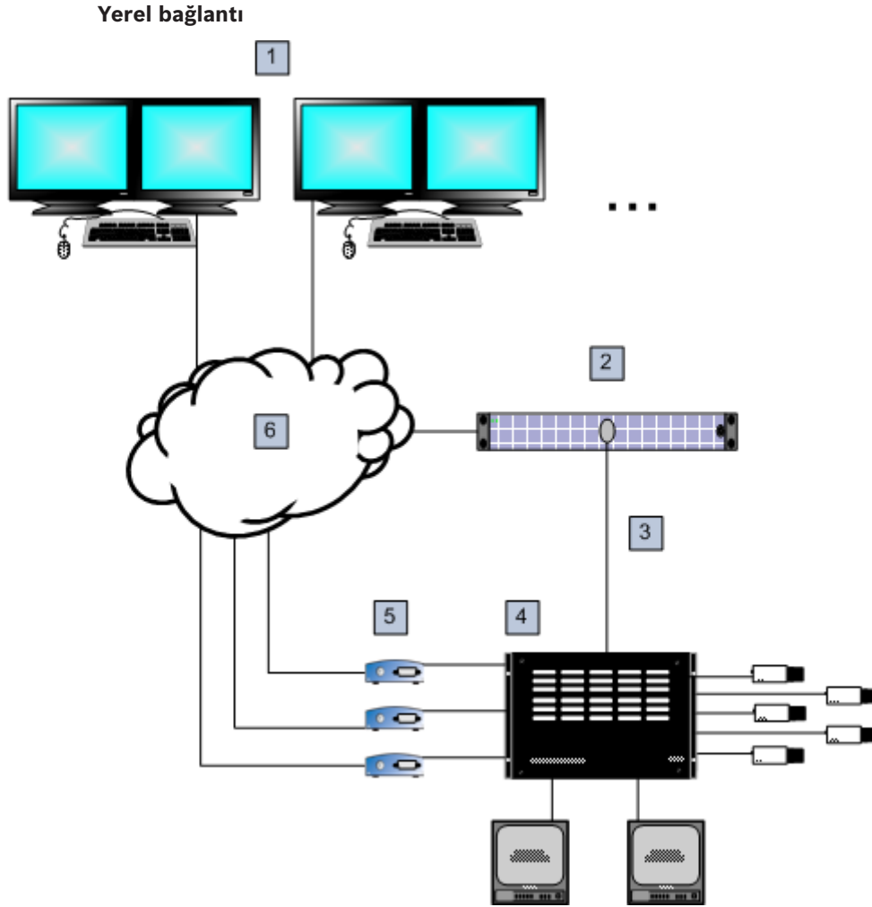
Şekil 5.3: Bosch Video Management System'in Bosch Allegiant matris anahtarına yerel bağlantısı
