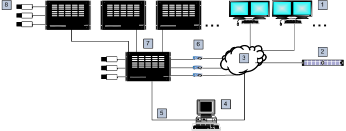
Şekil 5.5: Satellite anahtarlarıyla genişletilmiş Bosch Allegiant sistemi
