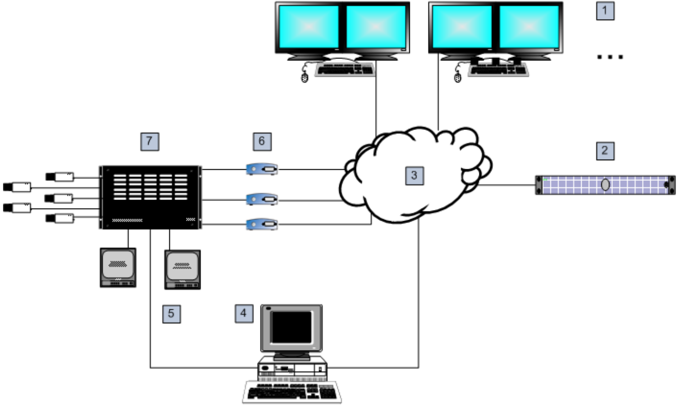
Şekil 5.4: Bosch Video Management System'in Bosch Allegiant matris anahtarına uzaktan bağlantısı
