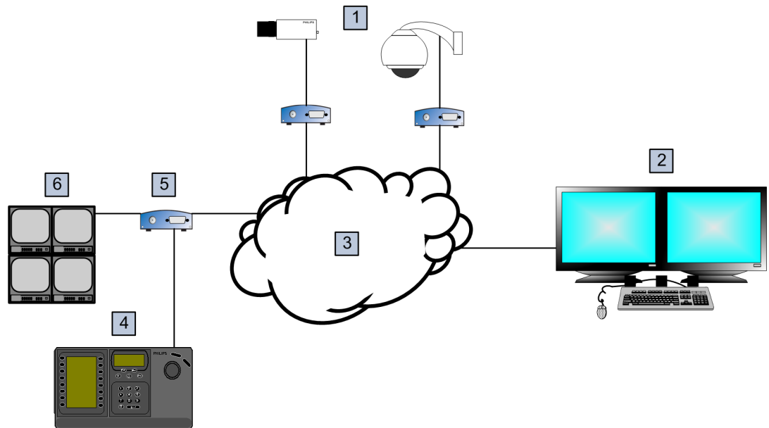
Afbeelding 5.2: Scenario 2: Bosch IntuiKey-bedieningspaneel aangesloten op een decoder
