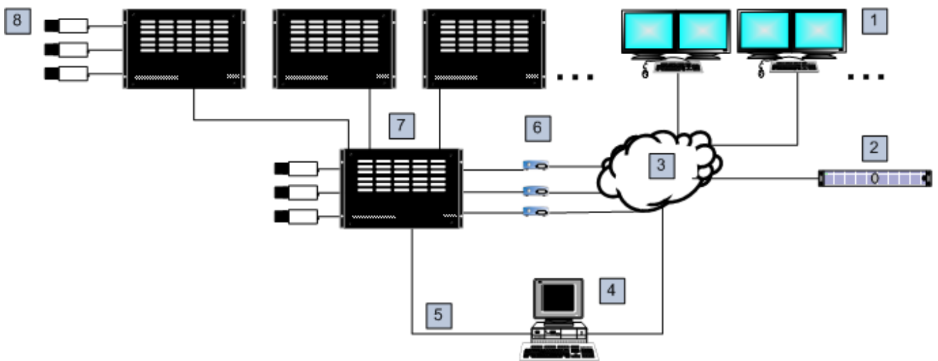
Afbeelding 5.5: Bosch Allegiant-systeem uitgebreid met satelliet-schakelaars
