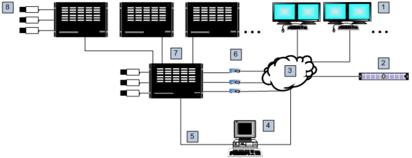
그림 5.5: 위성 스위치로 확장된 Bosch Allegiant 시스템
