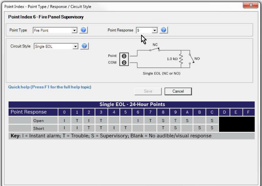
Figure 3.3: Réponse du type de point et type de circuit
