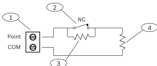
Figura 12.1: Cableado de entrada con resistencias de RFL duales
