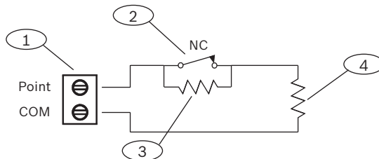
Figura 18.2: Cableado de entrada con resistencias de RFL duales
