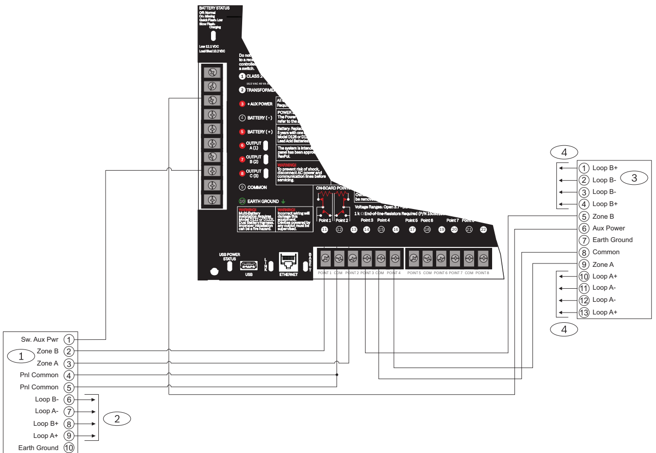
Figura 18.1: Cableado de entrada con un D125B y un D129
