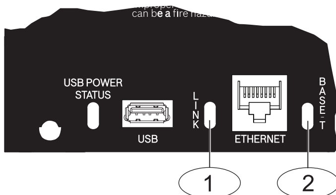
Figura 8.1: Ethernet y LED integrados en placa
