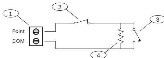
Figura 18.3: RFL única (NC o NA)
