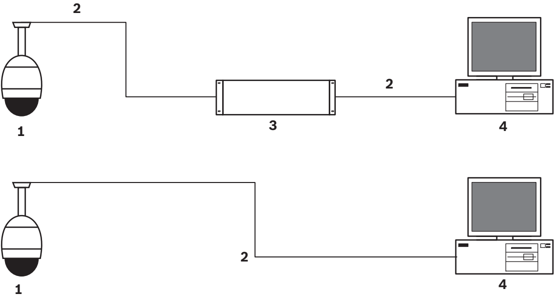
图 10.1: AUTODOME IP 系统配置
