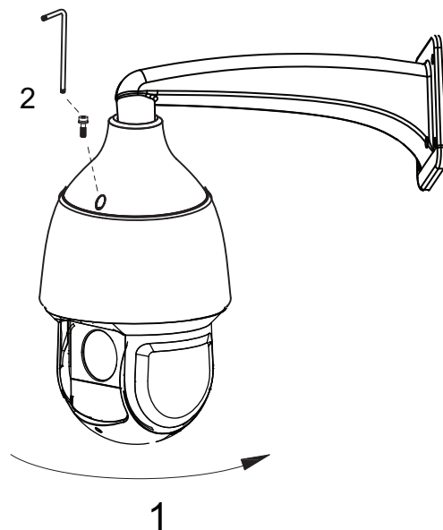
图 8.4: 将摄像机固定到底座
