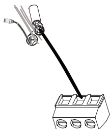
图 8.3: 穿过墙壁底座的缆线
