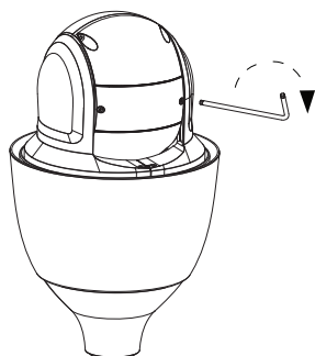
图 7.5: 拧紧螺丝
