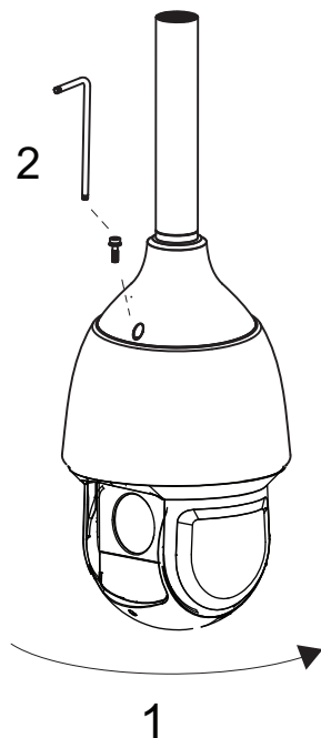
图 9.1: 将摄像机固定到底座
