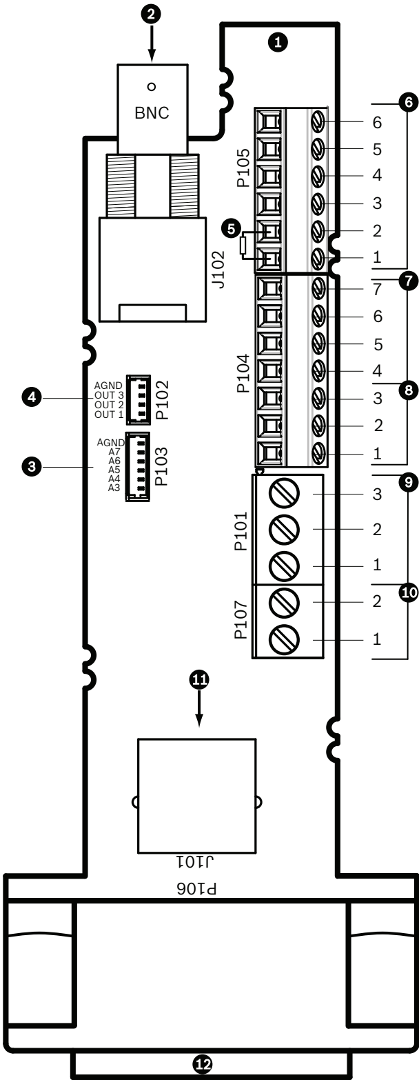
图 8.11: 管道接口板连接
