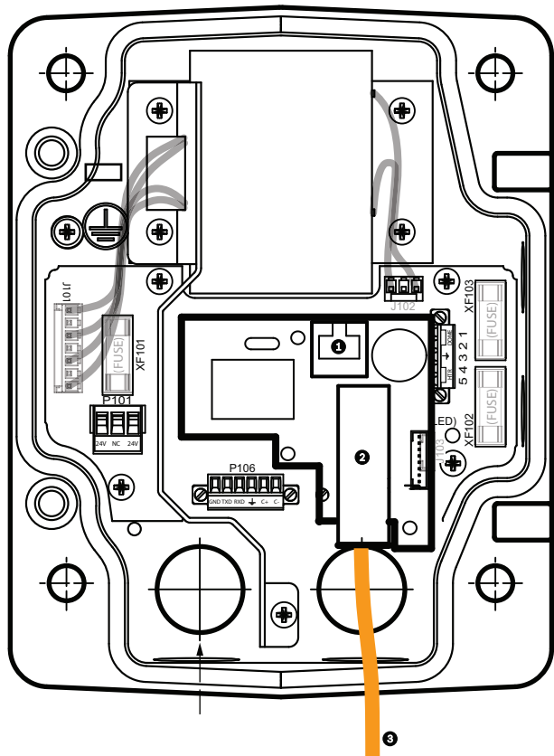
图 8.3: 已安装光纤以太网模块
