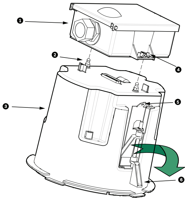
图 9.10: 嵌入天花板式防护罩和接口盒
