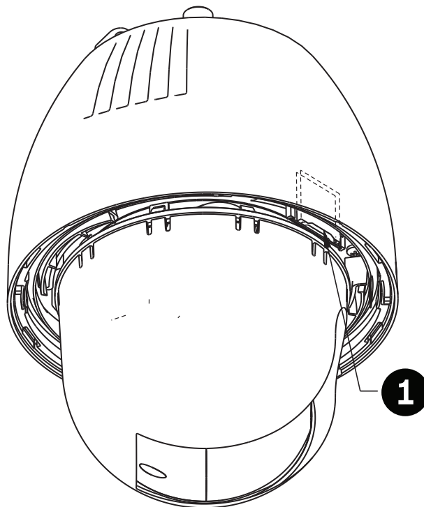
图 5.1: 带有 SD 卡插槽的摄像机横截面
