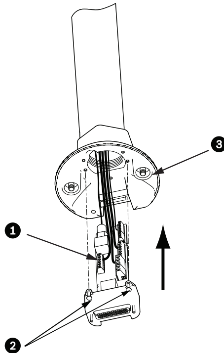
图 8.13: 装配管道接口板与球型顶盖
