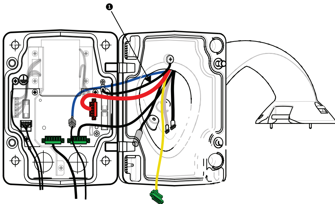
图 7.8: 连接吊装臂与电源盒
