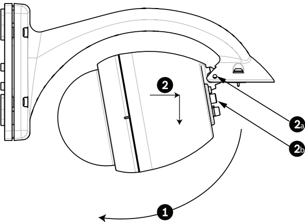
图 7.12: 连接吊装件到吊装臂
