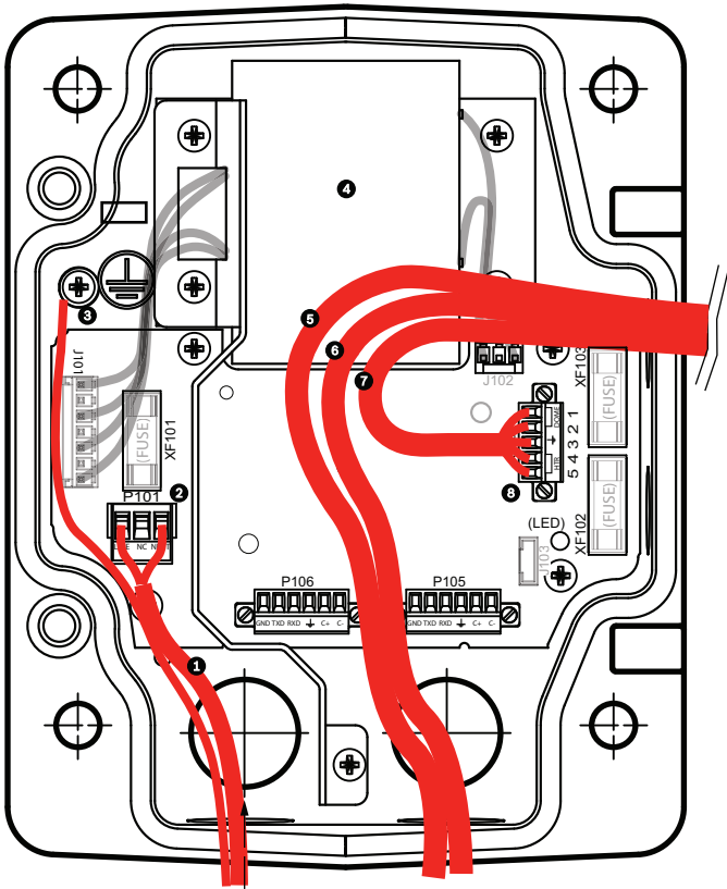
图 8.1: VG4-A-PSU1 或 VG4-A-PSU2 电源盒
