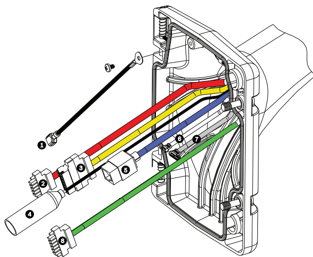
图 7.10: 吊装臂缆线
