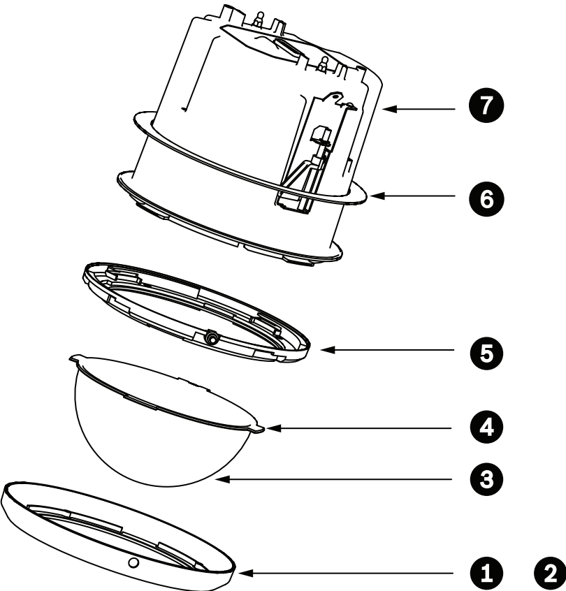
图 9.8: 嵌入天花板式 (符合 IP54 防护等级标准) 安装图
