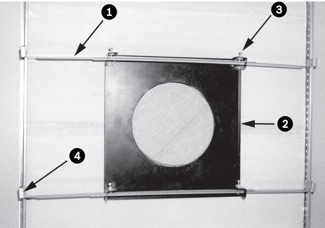
图 9.1: 吊顶天花板支架 (俯视图)
