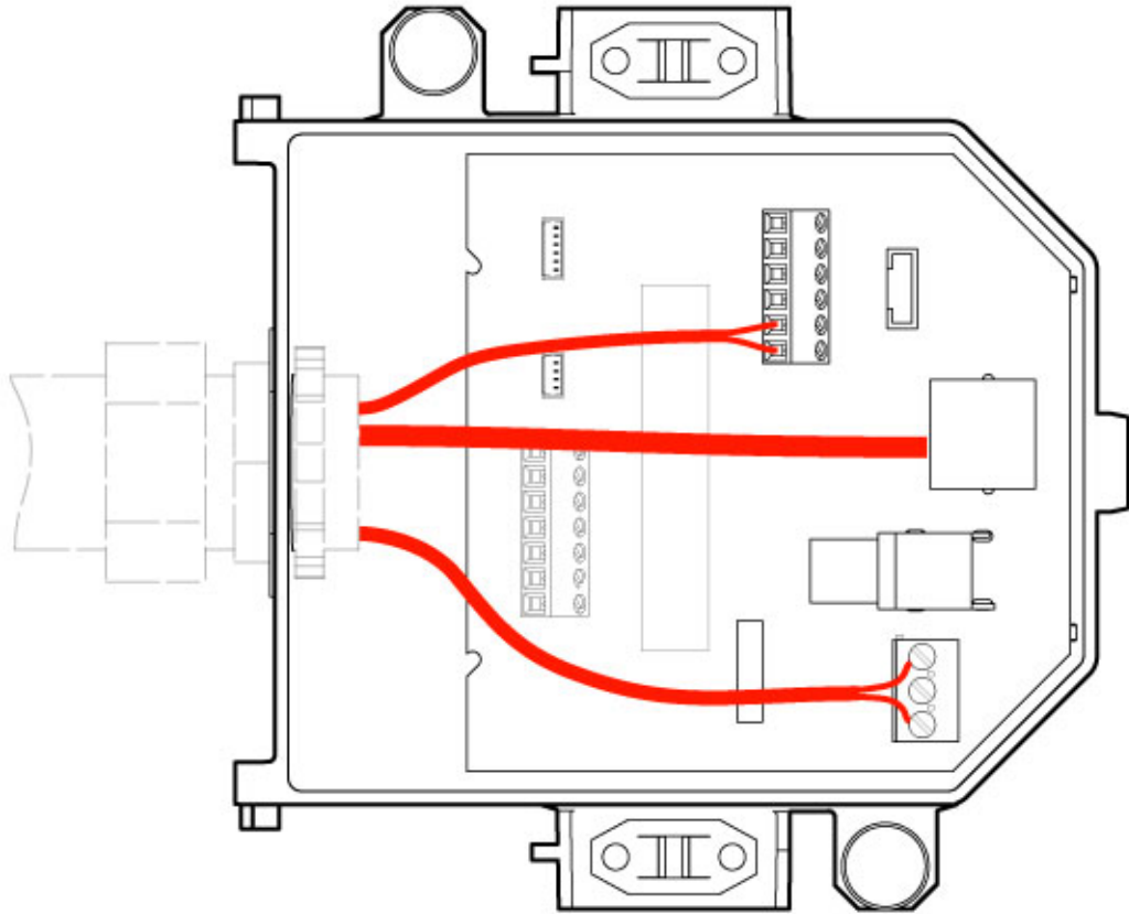
图 9.5: 接口盒连接
