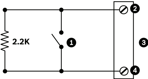
图 11.2: N.O.S. - 常开受监测连接
