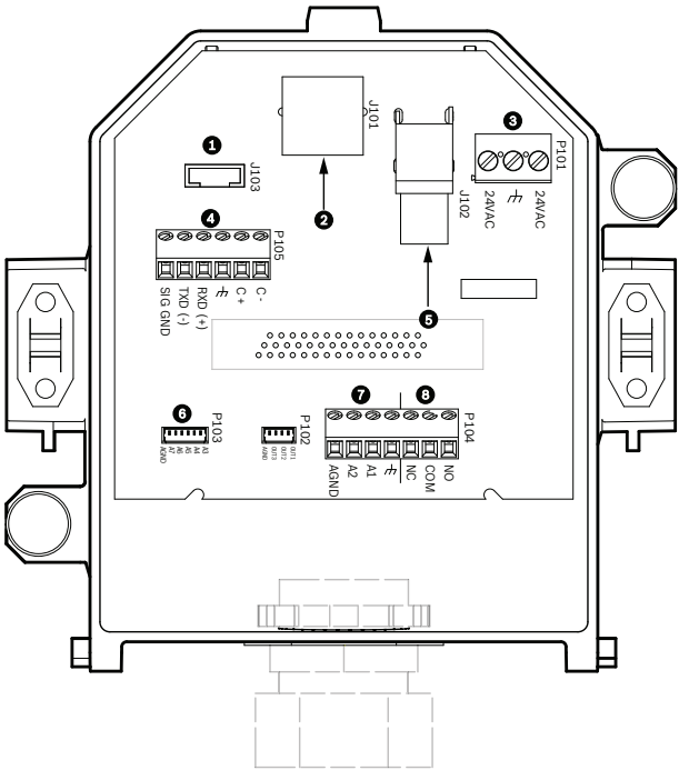
图 9.7: 嵌入天花板式接口盒
