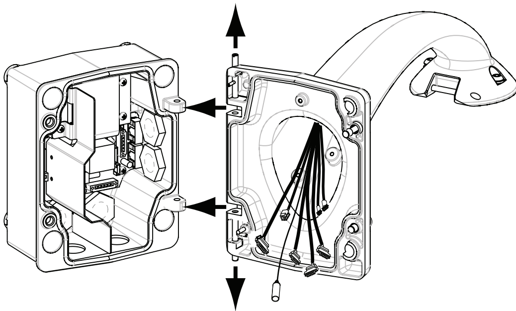
图 7.7: 对齐吊装臂与电源盒铰链接口
