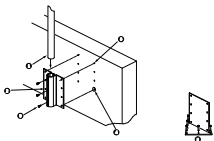
图 8.7: 护栏墙壁底座支架和屋顶底座板
