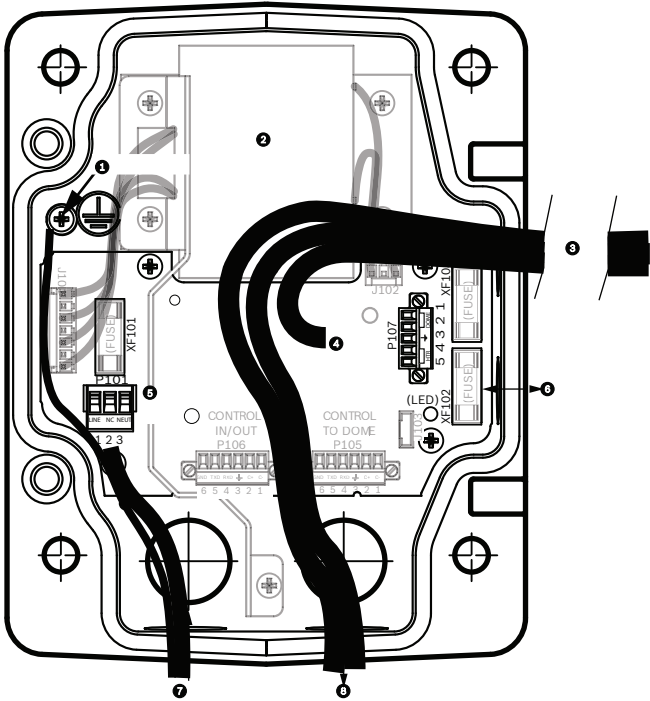
图 8.4: 电源盒连接
