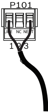
图 7.4: 引入的 115/230 VAC 电源
