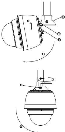
图 8.14: 吊装件与屋顶/管道底座的连接
