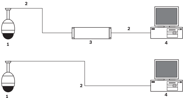
图 11.1: AUTODOME 7000 系列系统配置
