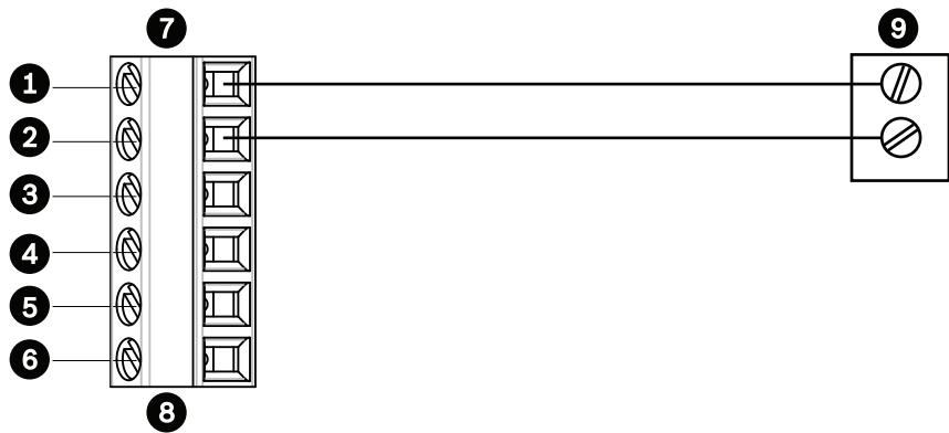
图 11.6: 通过以太网连接音频
