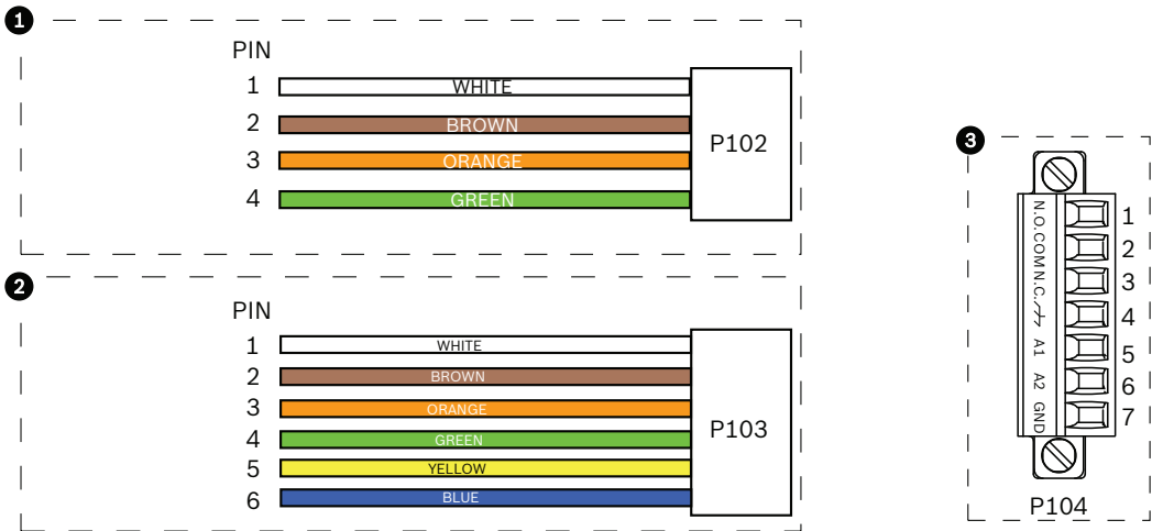
图 7.1: 报警和继电器连接器
