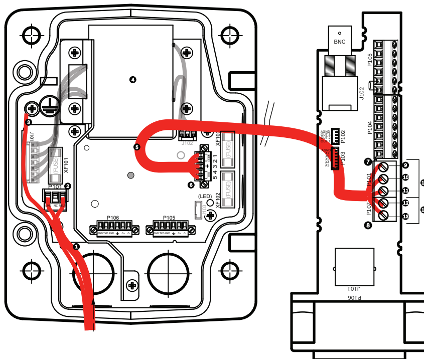
图 8.2: 连接至管道接口板的 VG4-A-PSU1 或 VG4-A-PSU2 电源盒
