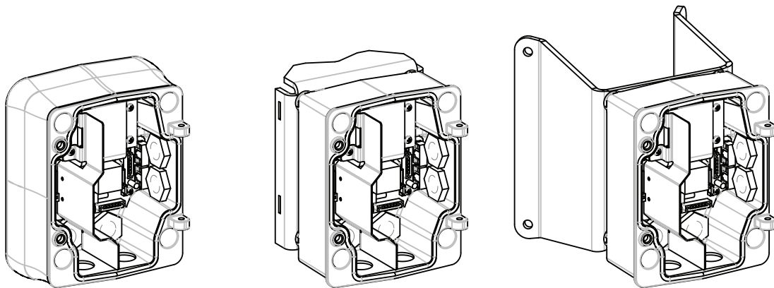
图 6.1: 电源设备的墙壁、立杆和角落底座
