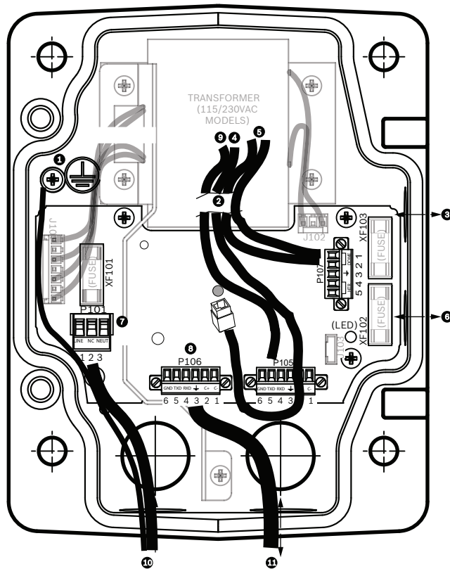
图 7.2: 吊装臂电源盒
