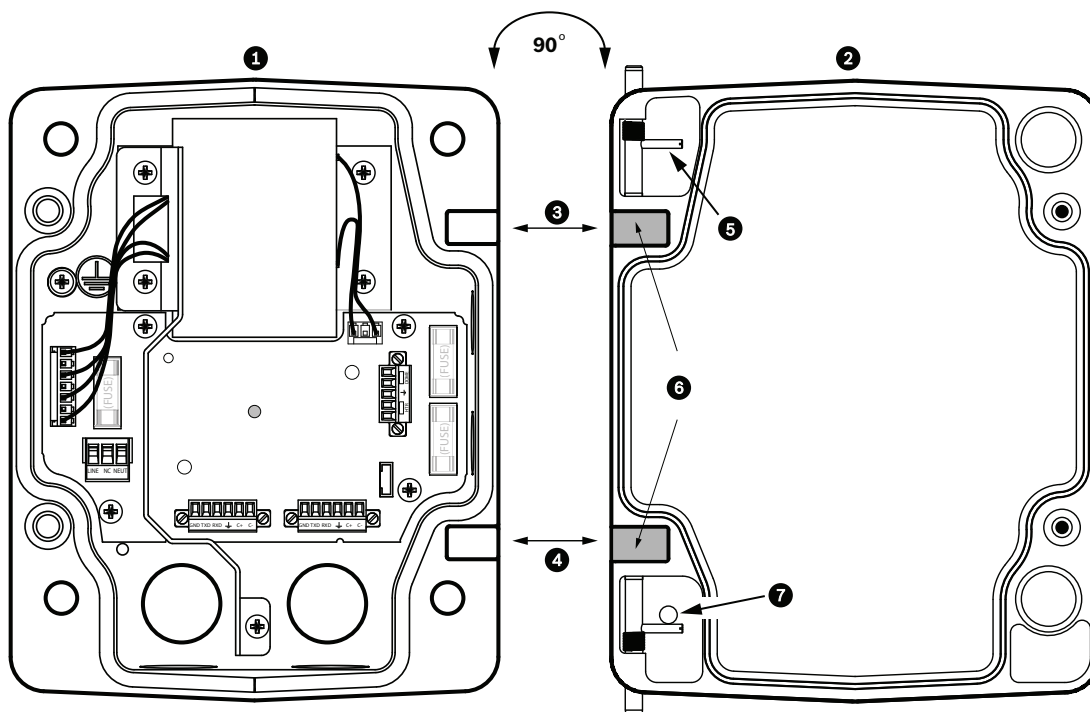
图 8.5: 对齐盖门铰链与电源盒
