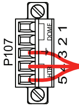
图 7.5: 引出的 24 VAC 电源
