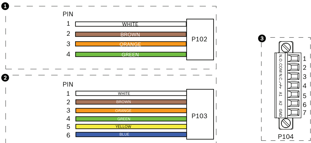
图 8.12: 报警和继电器连接器
