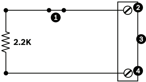
图 11.3: N.C.S. - 常闭受监测连接
