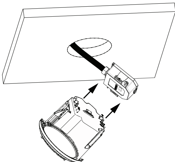
图 9.9: 将防护罩连接至接口盒
