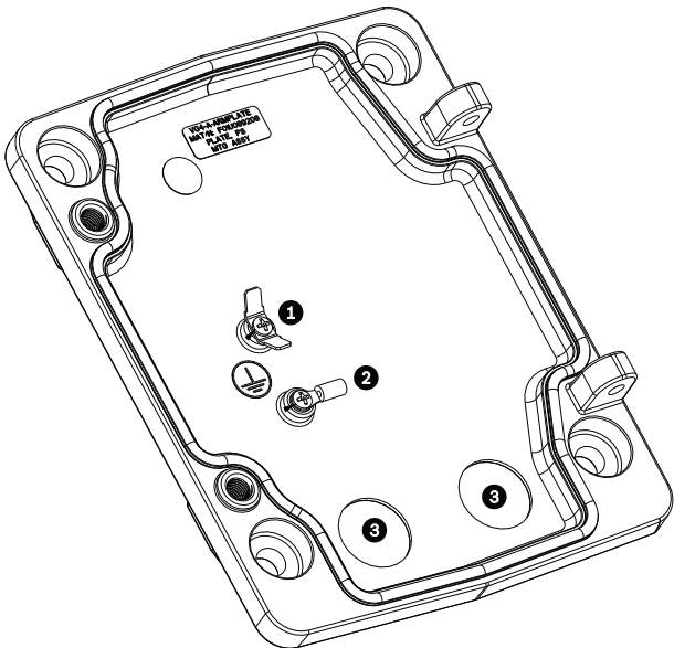
图 7.11: 安装板 - 内部细节
