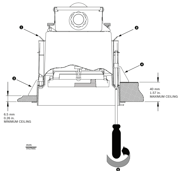
图 9.11: 将摄像机固定到天花板
