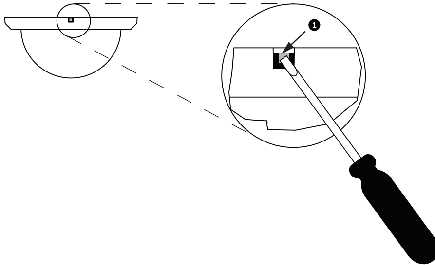
图 10.1: 球型罩释放螺丝
