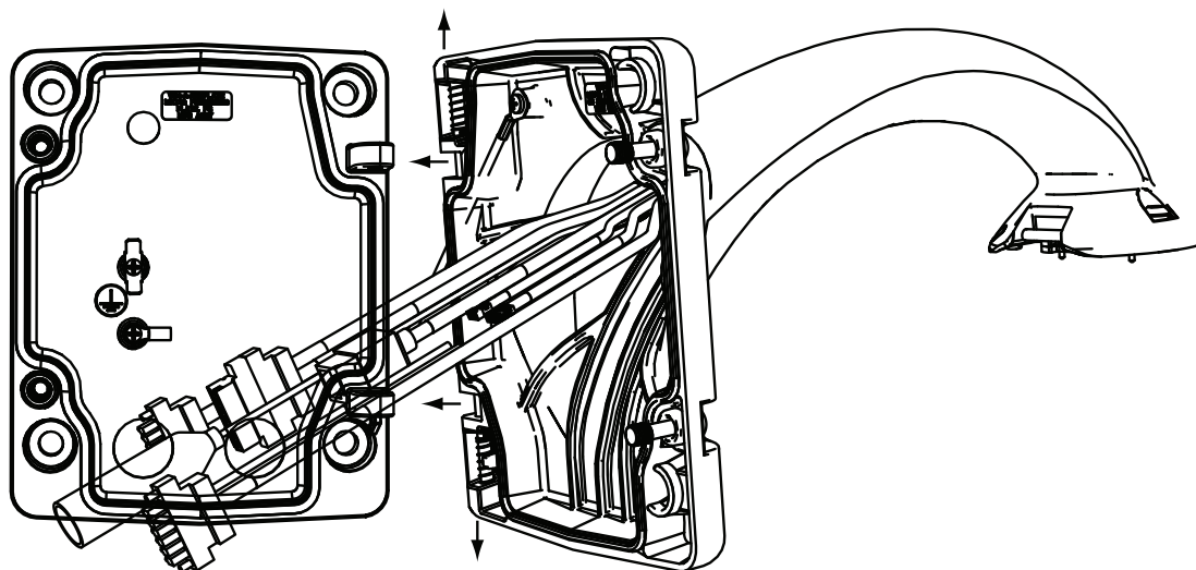
图 7.9: 将吊装臂连接到安装板
