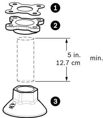
图 8.10: 管道底座
