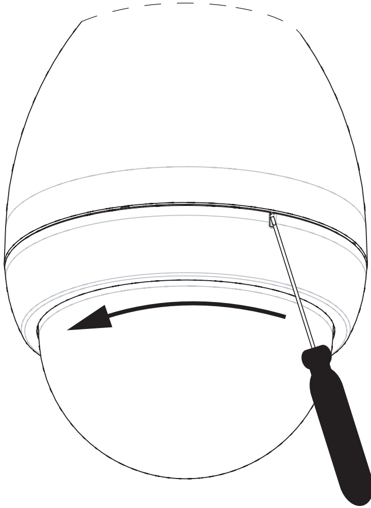
图 10.2: 吊装球型罩释放孔
