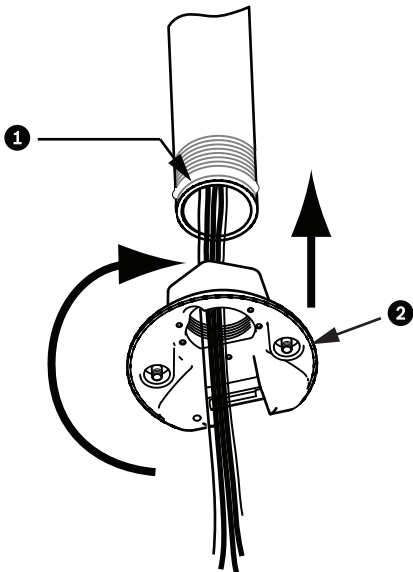
图 8.9: 连接球型顶盖
