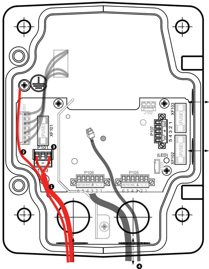
图 7.6: VG4-PA0 电源盒
