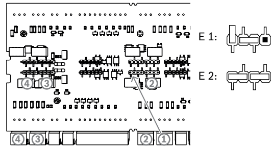
圖片 4.20: 繼電器輸出跨接線的位置 (底側)
