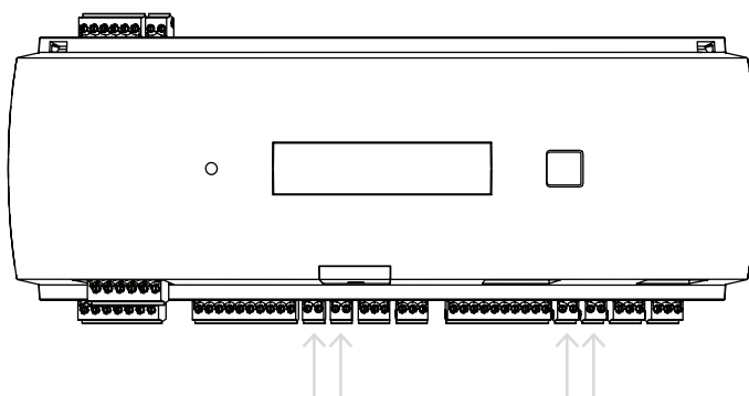
圖片 4.21: 類比輸入接頭的位置
