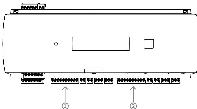
圖片 4.16: 供讀卡機使用的 Wiegand 介面 (連接埠) 位置
