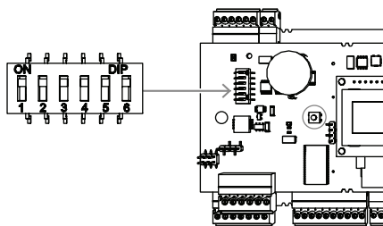
圖片 7.2: DIP 開關
