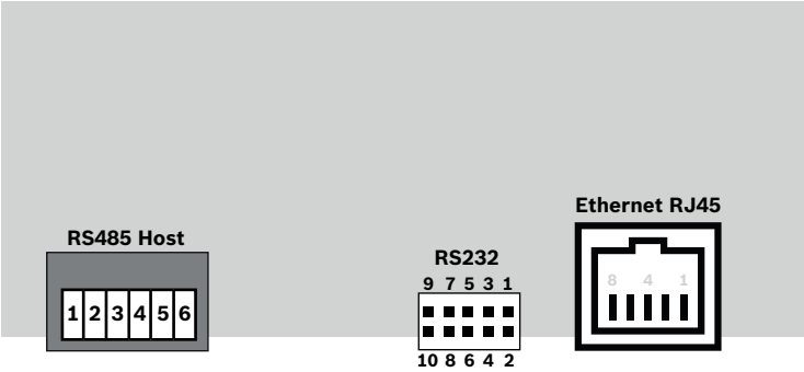
圖片 11.1: 上方 PCB 上的接頭 以下版本不支援 RS-485 介面: - BIS 4.9.1 及更新版本 - AMS 4.0 及更新版本。
