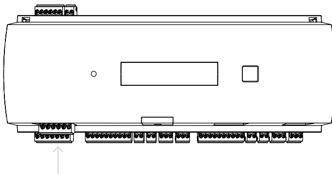
圖片 4.7: 電源供應器接頭的位置
