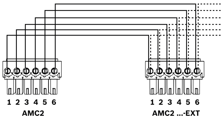
圖片 4.15: 擴充模組與控制器的連接
