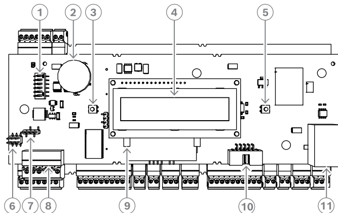
圖片 3.3: 上方電路板含顯示器 (正面)
