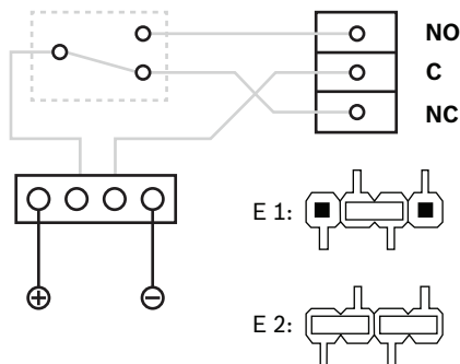
圖片 4.18: 繼電器模式設定
