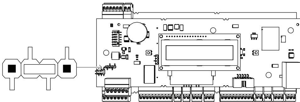
圖 4.12: RS 485 四線式連接的設定
