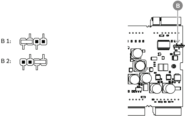
圖片 4.6: 接地跨接線底部的位置
