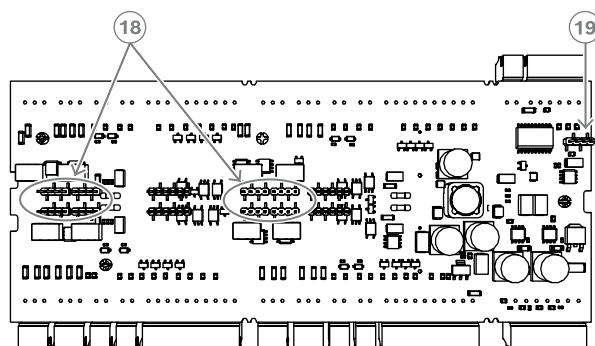
圖片 3.5: 跨接線 (背面)
