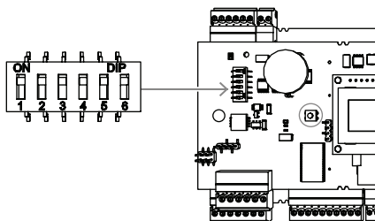
圖片 4.13: 主機設定切換裝置的位置
