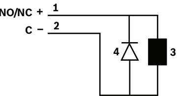
圖片 4.19: 復原二極體線路圖
