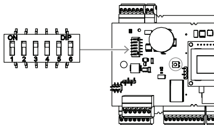
图片 7.2: DIP开关
