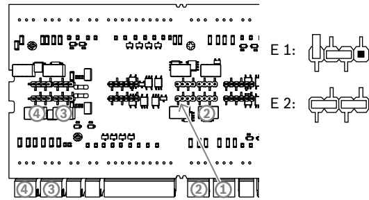
图片 4.20: 继电器输出跳线的位置（底部）
