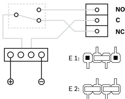
图片 4.18: 继电器模式设置
