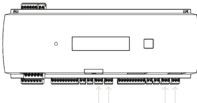
图片 4.17: 继电器输出连接器的位置
