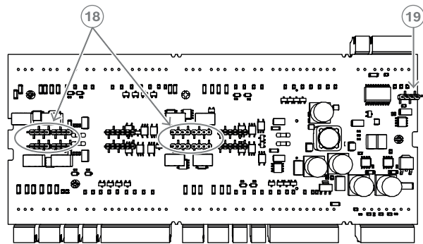
图片 3.5: 跳线（背面）
