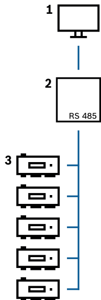
图片 4.9: RS-485主机系统的配置
