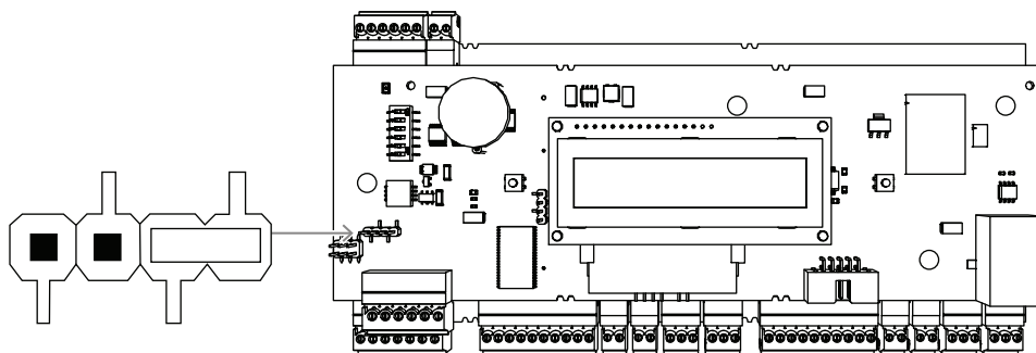
图片 4.11: RS-485 双线连接的跳线设置
