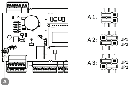
图片 4.5: 接地跳线RS-485主机接口的位置
