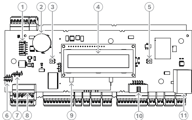
图片 3.3: 带显示屏的上部电路板（正面）
