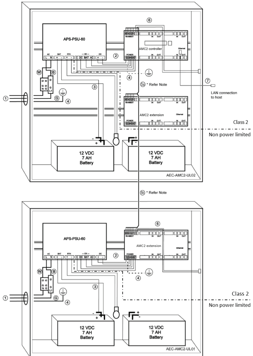
图片 6.1: 带扩展的安装示例
