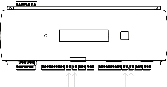
图片 4.21: 模拟输入连接器的位置
