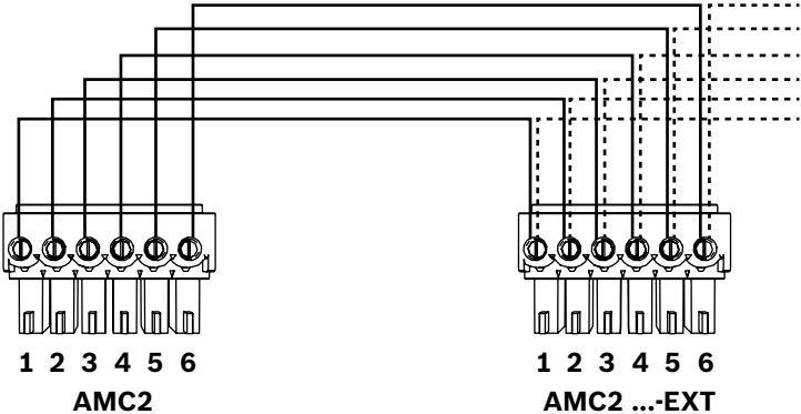
图片 4.15: 将扩展模块连接到控制器
