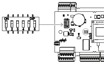
图片 4.13: 主机设置选择器的位置
