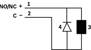
图片 4.19: 恢复二极管示意图
