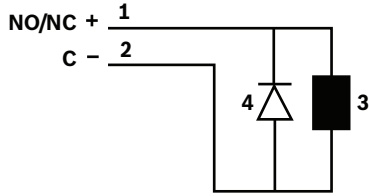
Şekil 4.19: Kurtarma diyotu şematiği
