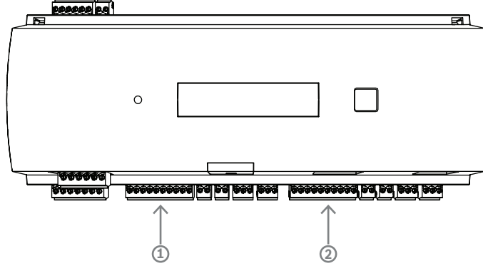
Şekil 4.16: Okuyuculara ait Wiegand arayüzünün (port) konumu
