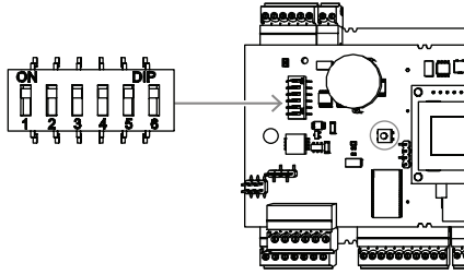
Şekil 4.13: Ana bilgisayar ayarları için seçicinin konumu
