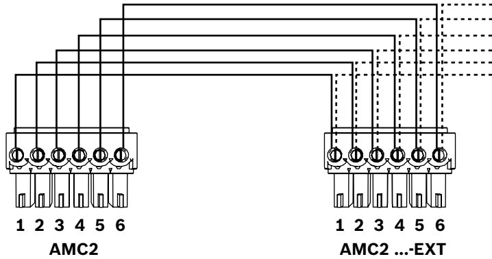
Şekil 4.15: Genişletme modülünün AMC2 bağlantısı
