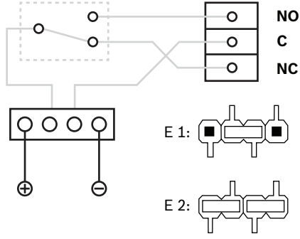
Şekil 4.18: Röle modu ayarları
