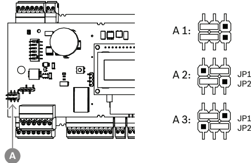
Şekil 4.5: RS-485 ana bilgisayar arayüzünün topraklama anahtarının konumu
