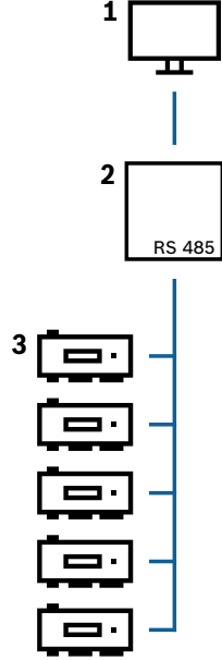
Şekil 4.9: RS-485 ana bilgisayar sisteminin yapılandırması
