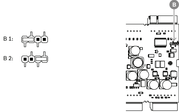
Şekil 4.6: Topraklama anahtarı alt tarafının konumu
