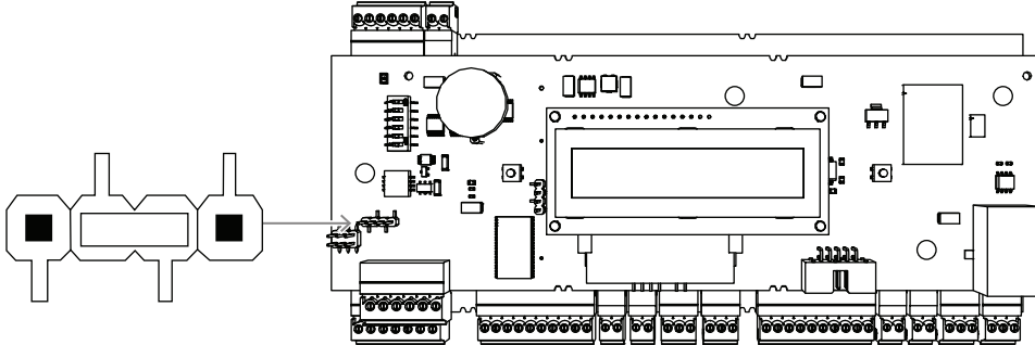
Şekil 4.12: RS-485 dört kablolu bağlantı ayarları
