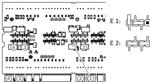
Şekil 4.20: Röle çıkış anahtarlarının konumu (alt taraf)
