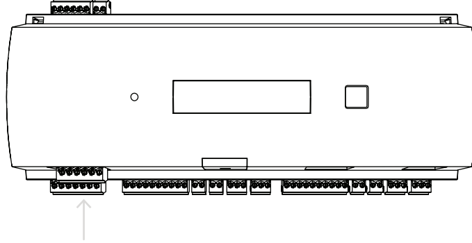
Şekil 4.7: Güç kaynağı konnektörünün konumu
