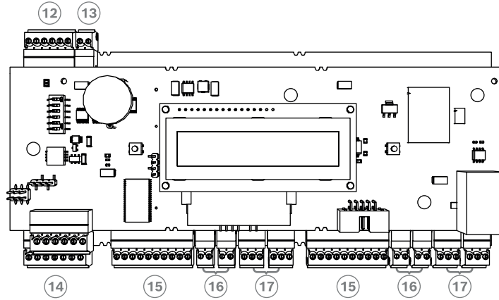
Şekil 3.4: Arayüzler - genel bakış
