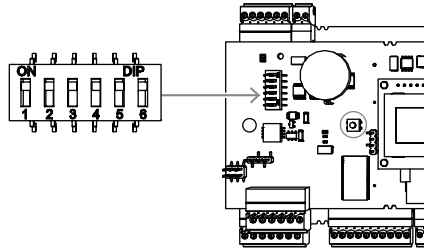
Şekil 7.2: DIP anahtarları
