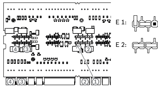
Рис. 4.20: Расположение перемычек релейных выходов (нижняя сторона)
