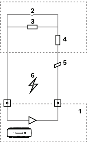
Рис. 4.22: Схема цепи
