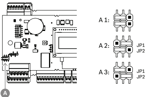
Рис. 4.5: Расположение перемычки заземления интерфейса RS-485 главного компьютера
