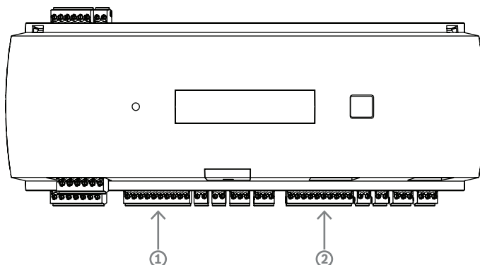
Рис. 4.16: Расположение интерфейса (порта) Wiegand для считывателей
