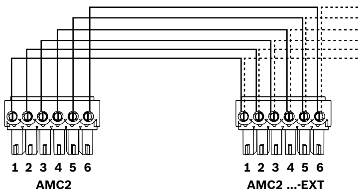
Рис. 4.15: Подключение модуля расширения к контроллеру
