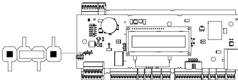
Рис. 4.12: Настройки для четырехпроводного подключения RS-485
