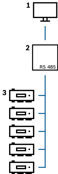
Рис. 4.9: Настройка главной системы RS-485
