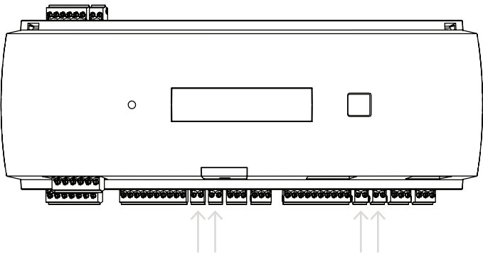
Рис. 4.21: Расположение разъемов аналоговых входов
