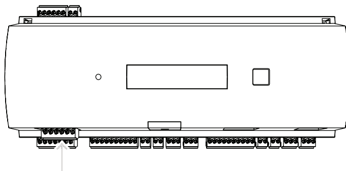
Рис. 4.10: RS-485-интерфейс сервера
