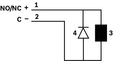
Рис. 4.19: Схема восстановительных диодов
