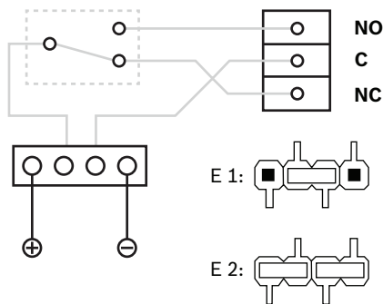
Рис. 4.18: Настройки режима реле
