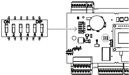
Рис. 4.13: Расположение селектора для настройки параметров сервера
