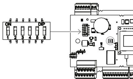
Рис. 7.2: DIP-переключатели
