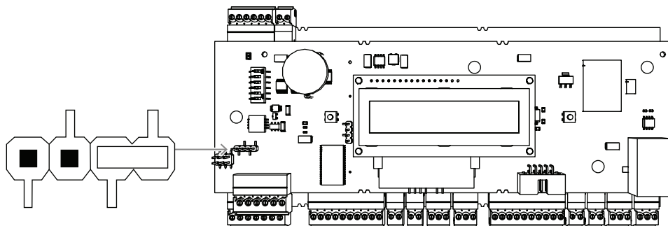
Рис. 4.11: Настройка перемычек для двухпроводных подключений RS-485
