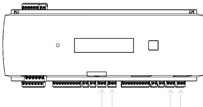
Afbeelding 4.17: Locatie van de relaisuitgangs-aansluitklemmen
