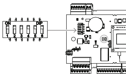
Afbeelding 7.2: DIP-schakelaars
