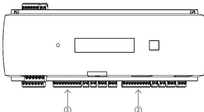
Afbeelding 4.16: Locatie van de Wiegand-interface (poort) voor lezers
