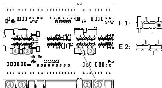
Afbeelding 4.20: Locatie van jumpers voor de relaisuitgangen (onderkant)
