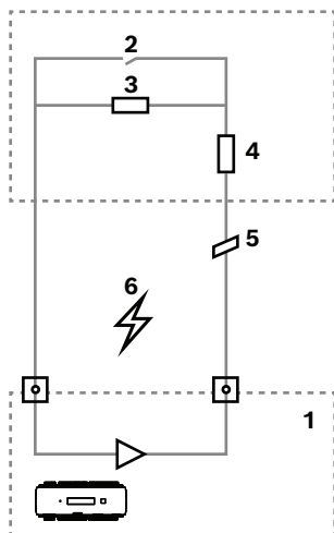
Afbeelding 4.22: Schakelschema
