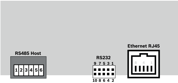
Afbeelding 11.1: Aansluitklemmen op de bovenste PCB De RS-485 interface wordt niet ondersteund door: – BIS 4.9.1 en hoger – AMS 4.0 en hoger.
