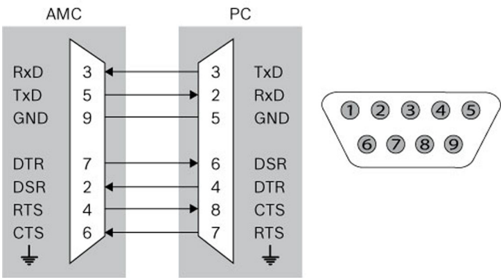
Afbeelding 11.2: Onderling verbindingsdiagram van de projectspecifieke interface
