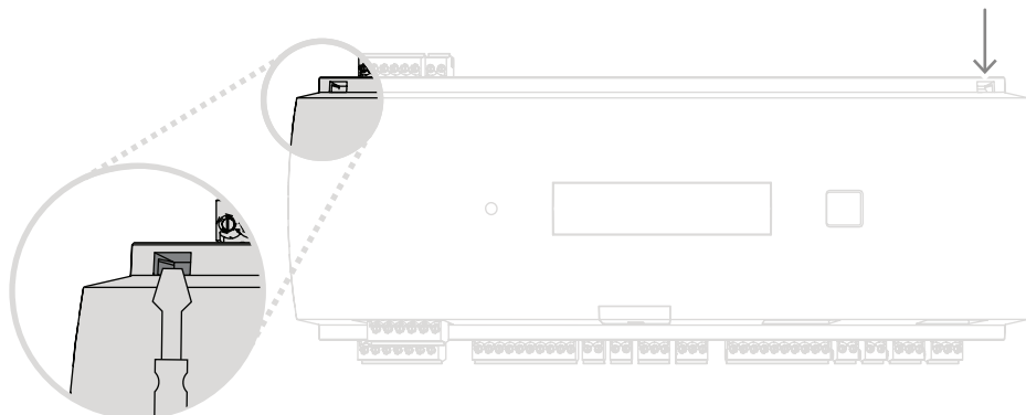
Afbeelding 4.3: De behuizing van de controller openen
